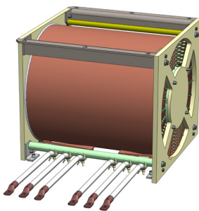
Stabkerndrossel SD
