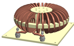
Luftdrossel TD
